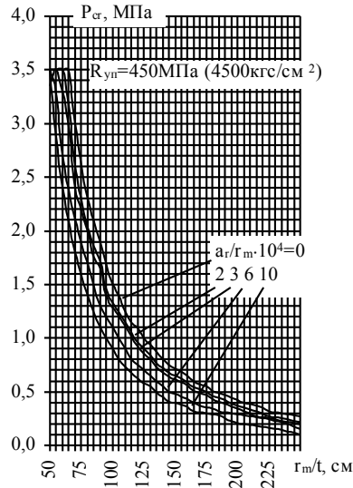
Черт. 2. График зависимости критического наружного давления p_{cr} от относительной толщины стенки r_m/t [ R_{yn} – нормативное сопротивление по пределу текучести стали, МПа (кгс/см 2 ); a_r – расчетный радиальный зазор между стенкой оболочки и бетоном, см; r_m – средний радиус оболочки, см; t – толщина стенки оболочки, см]
