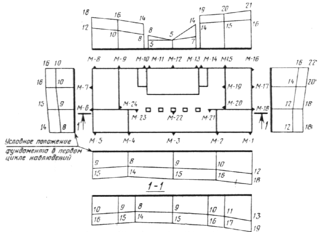
График давления на основание фундамента
