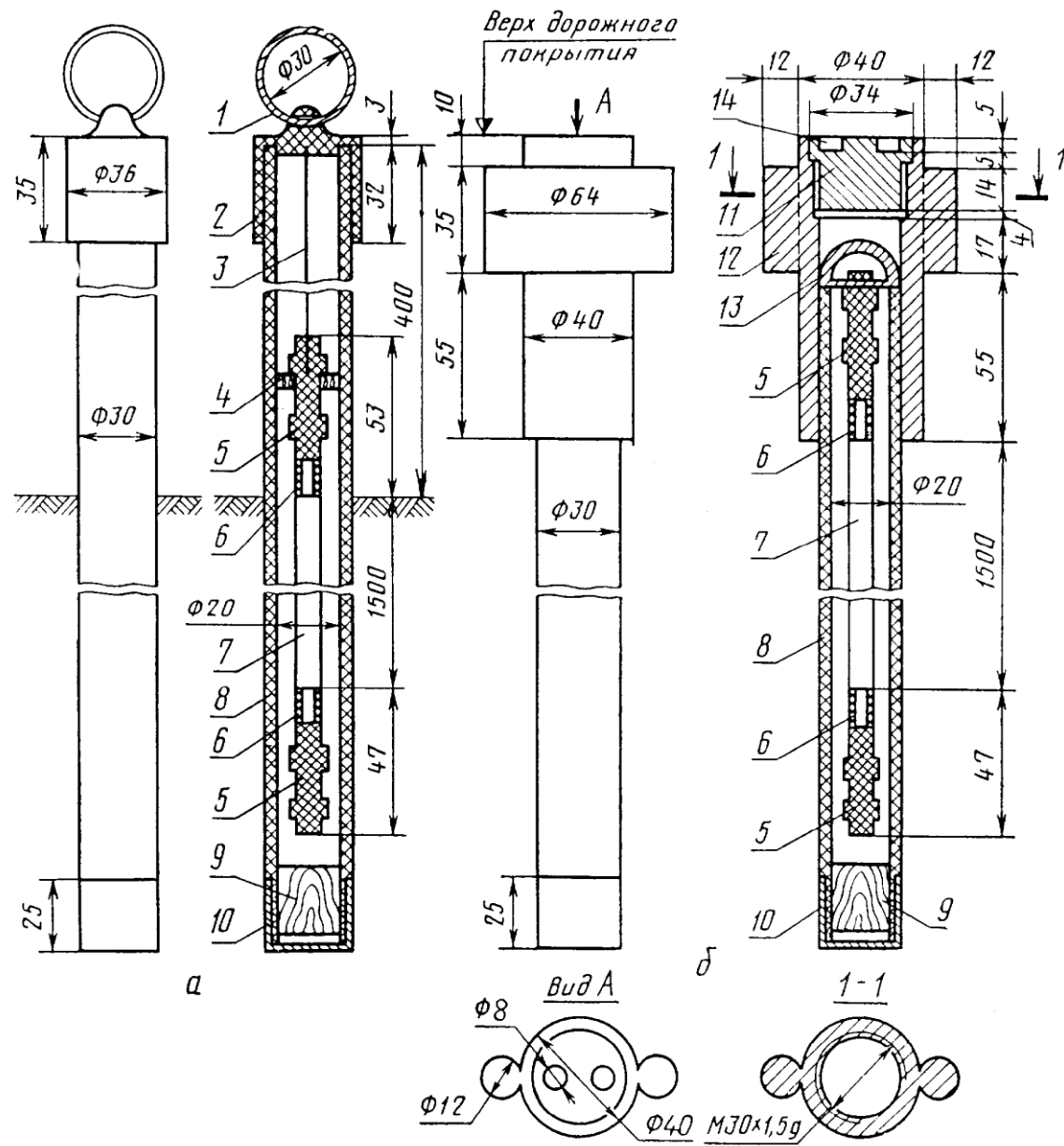
а - общий вид и продольный разрез мерзлотомера, устанавливаемого на поверхности рельефа; б - то же, устанавливаемого заподлицо с
