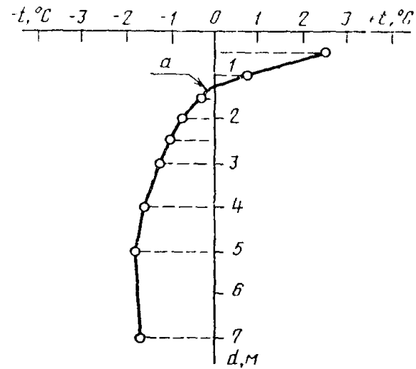
График распределения температуры t , °C, грунта по длине d , м, для одноразовых измерений температуры
