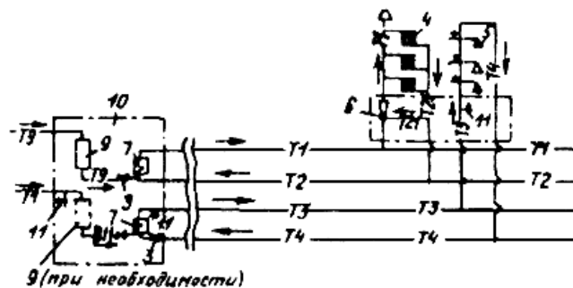
Рис.3. Схема теплоснабжения с отдельными сетями горячего водоснабжения
