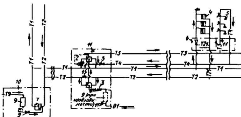
Рис. 1. Схема закрытой системы теплоснабжения
