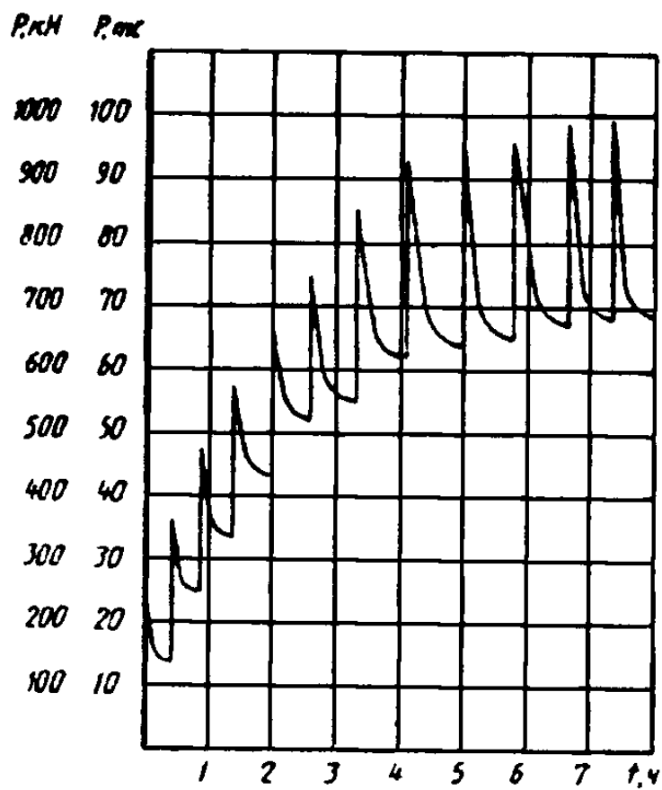
Рисунок 2 - График релаксации нагрузки за время испытания
