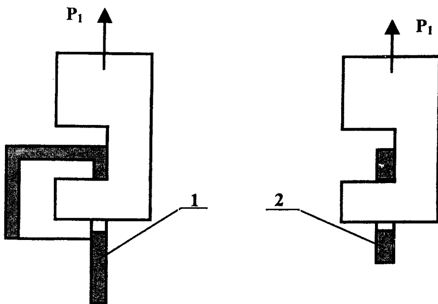
Рисунок 4 — Схема испытаний силой P_1 запирающих планок накладного замка (1) и врезного замка (2)
