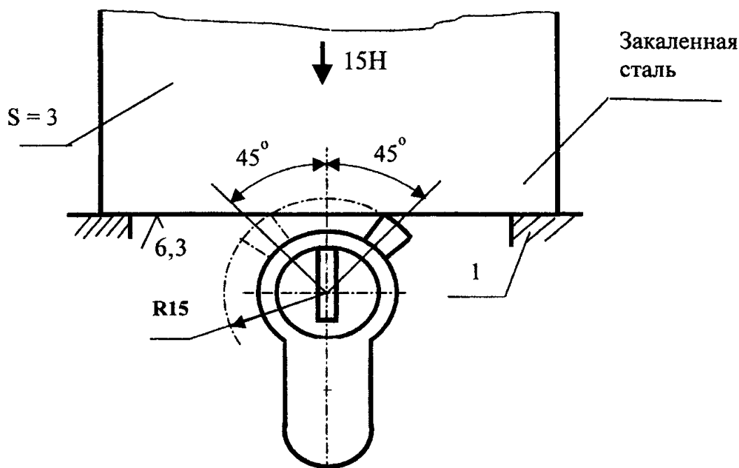
Рисунок 1 — Схема испытания цилиндрического механизма на наработку
