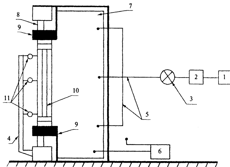
1 — компрессор (воздушный насос); 2 — регулятор расхода воздуха; 3 — запорный кран; 4 — приспособление для крепления измерительных приборов; 5 — шланги; 6 — датчики давления (манометры); 7 — герметичная камера; 8 — приспособление для крепления образца; 9 — эластичные уплотняющие прокладки; 10 — образец; 11 — измерительные приборы (например, цифровые индикаторы)
