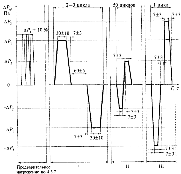
Рисунок 2 — Пример построения графиков испытаний
