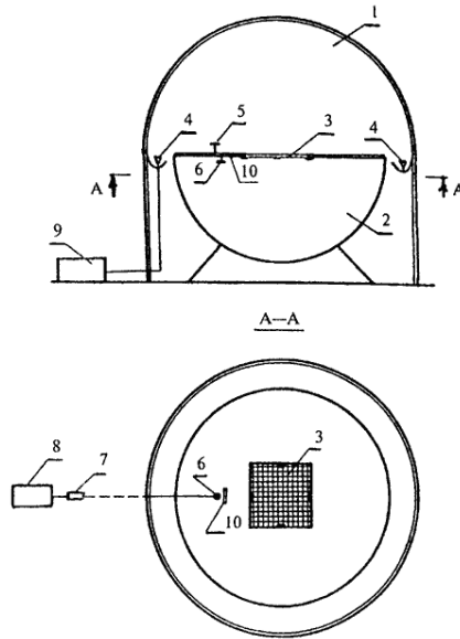
1 — источник диффузного света; 2 — светомерная камера; 3 — проем с опорной решеткой; 4 — осветительные приборы источника света; 5 — наружный фотоэлемент; 6 — внутренний фотоэлемент; 7 — переключатель фотоэлементов; 8 — микроамперметр или гальванометр; 9 — регулятор напряжения осветительных приборов; 10 — экран фотоэлемента от прямого света источника
