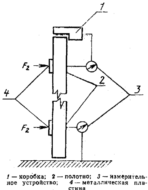
Рисунок 4 — Схема измерения перемещений под нагрузкой F_2
