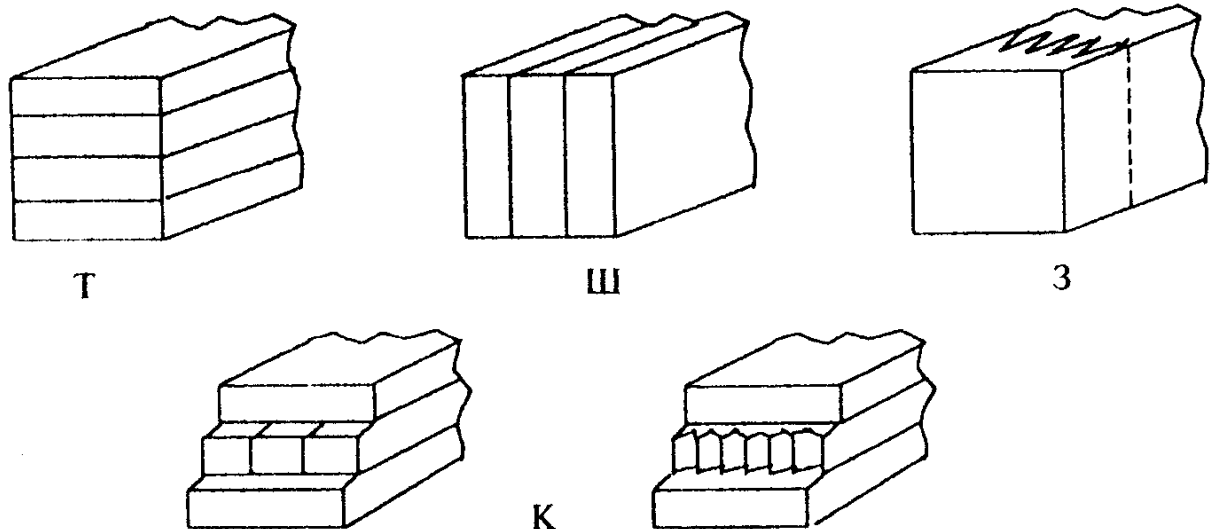
Рисунок 1 — Примеры схем склеивания
