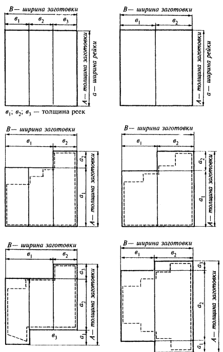
А; В; a_1 ; a_2 ; a_3 ; \theta_1 ; \theta_2 ; \theta_3 — контролируемые размеры Рисунок 2 — Примеры сечений двух- и трехслойных брусовых заготовок для оконных блоков по ГОСТ 24700
