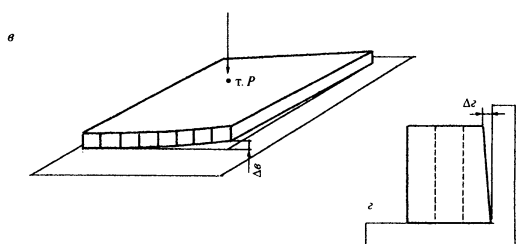
а — измерение отклонений от прямолинейности сторон, \Delta a ; б — измерение отклонений от плоскостности брусковых деталей и заготовок, \Delta a' ; в — измерение отклонений от плоскостности щитовых заготовок, \Delta b ; z — измерение отклонений от взаимной перпендикулярности сторон, \Delta z .
