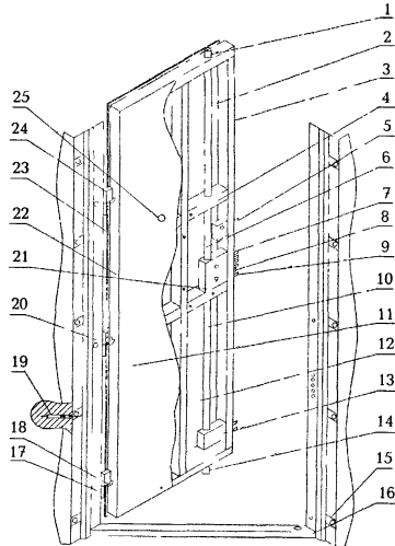
1 — верхний запирающий ригель, 2 — верхняя тяга основного замка, 3 — каркас полотна (сваренные стальные профили), 4 — места крепления внутреннего «лючка», 5 — задвижка, 6 — место крепления верхней тяги, 7 — ригели засова сувальдного замка, 8 — защелка, 9 — засов цилиндрического замка, 10 — нижняя тяга основного замка, 11 — места крепления отделки, 12 — внутренняя полость для наполнителя, 13 — направляющая вертикальной тяги, 14 — нижний запирающий ригель, 15 — монтажное «ушко», 16 — порог, 17 — отверстие под противосъемный ригель (штырь), 18 — противосъемный пассивный ригель (штырь), 19 — монтажный анкер, 20 — коробка (рама), 21 — комбинированный сувальдно-цилиндрический замок, 22 — внутренний стальной лист, 23 — наружный стальной лист, 24 — петлевой узел, 25 — глазок Рисунок 1 — Пример конструкции дверного блока, полотно которого сварено из двух стальных листов и стальных профилей, коробка (рама) — из стального гнутого профиля
